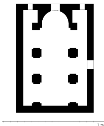
3.9. ზღუდერის ბაზილიკის გეგმა (პ. წუცუბიძის მიხედვით)
