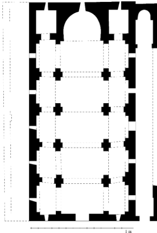
3.3. ურბნისის სიონის გეგმა (ა. სხვიტარიძე)
