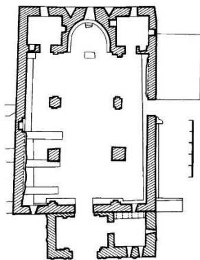
3.13. რკონის ბაზილიკის გეგმა (საქართველოს ისტორიისა და კულტურის ძეგლთა აღწერილობა, ტომი V. თბილისი, 1990.)
