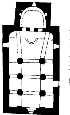
3.7. წუნისის ბაზილიკის გეგმა (რ. გვერდწითელის მიხედვით)
