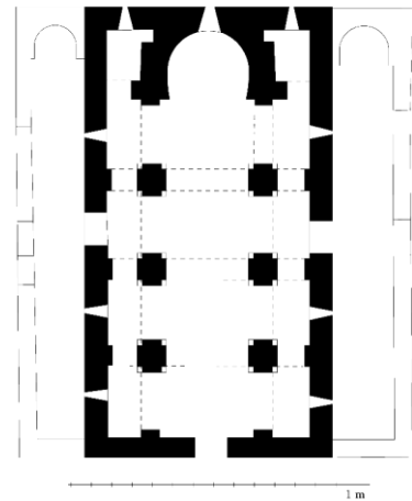
3.5. ნატკორას ბაზილიკის გეგმა (ა. სხვიტარიძე)
